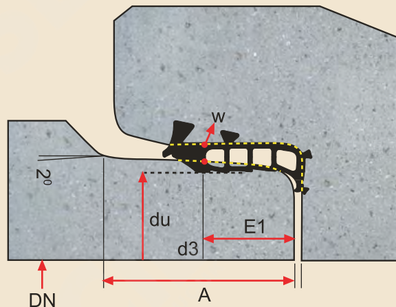
Entegre Contalı Boru Birleşim Detayı
