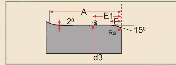
Şekil 4: Dış Fiber Başlığı Kesit ve Ölçüleri
