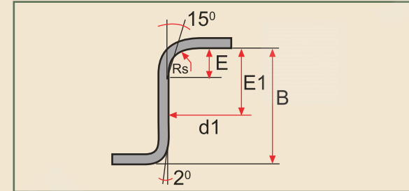
Şekil 4: Dış Fiber Başlığı Kesit ve Ölçüleri
