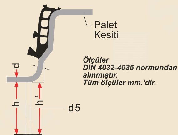
Entegre Contanın Palettaki Yerleşimi
